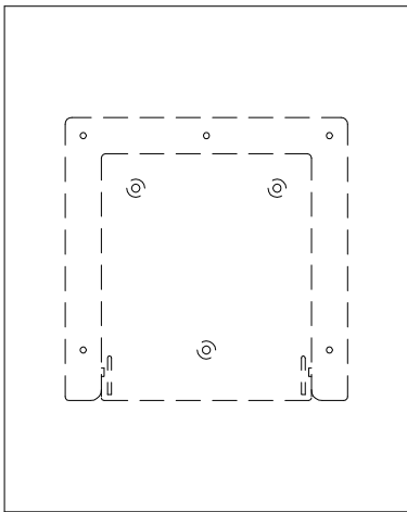
※スライドロック機構 脱着式 (ABS樹脂成形)
