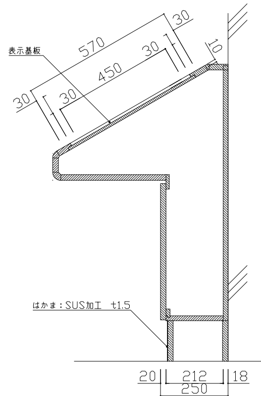
断面図
