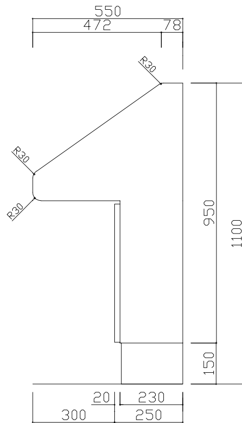
側面図
