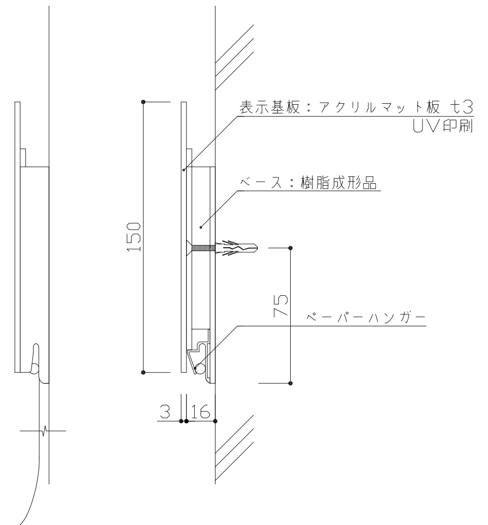
< 側面図 >
