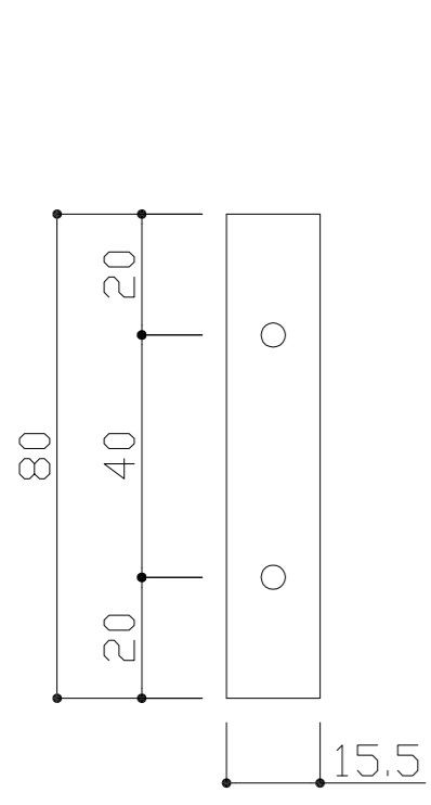
※取付ビス位置
