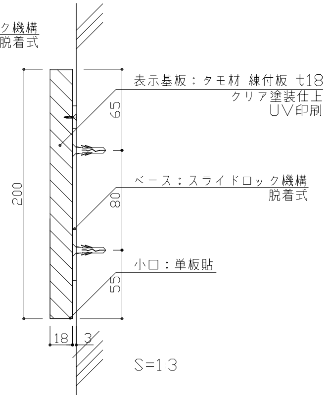
※スライドロック機構 脱着式 (ABS樹脂成形)
