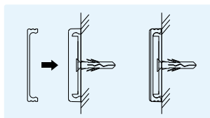
取付断面図
