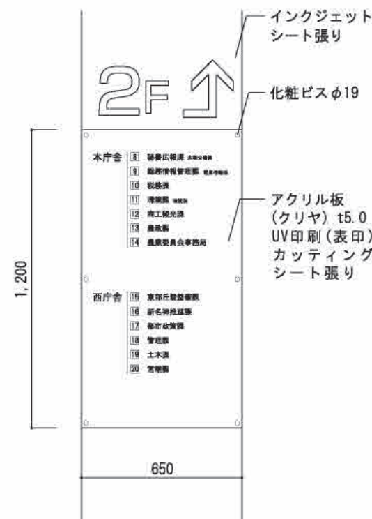
<柱(F通り・8通り) 東面>
