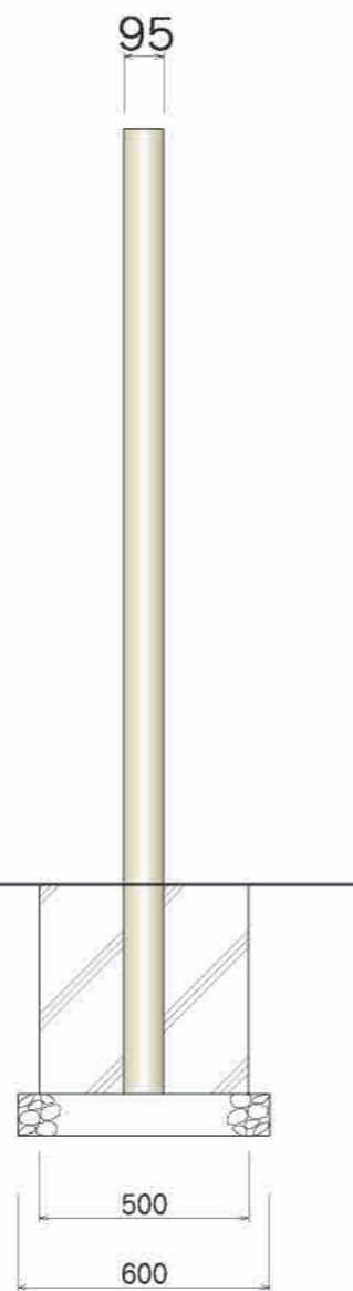
【側面図 S=1:20】
