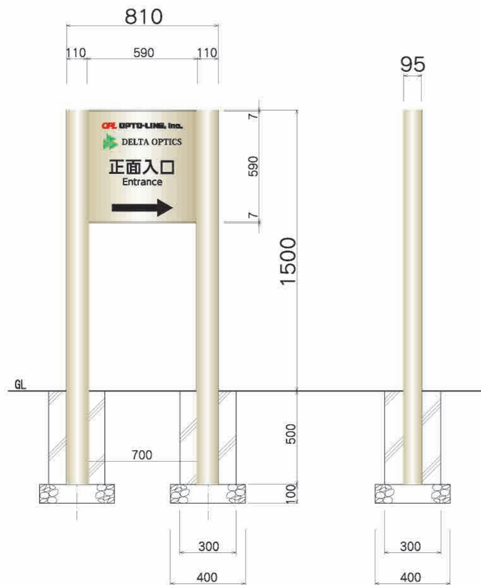
【正面図 S=1:20】
