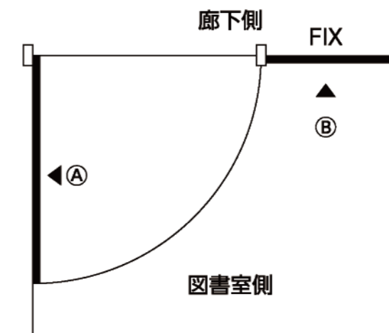
取付配置図
