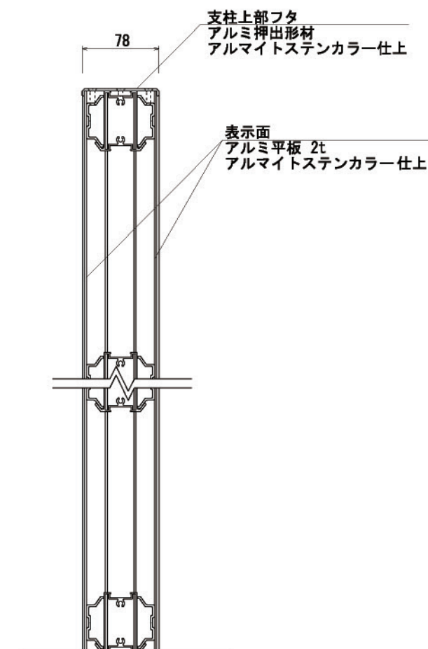
【側断面図 S=1:5】
