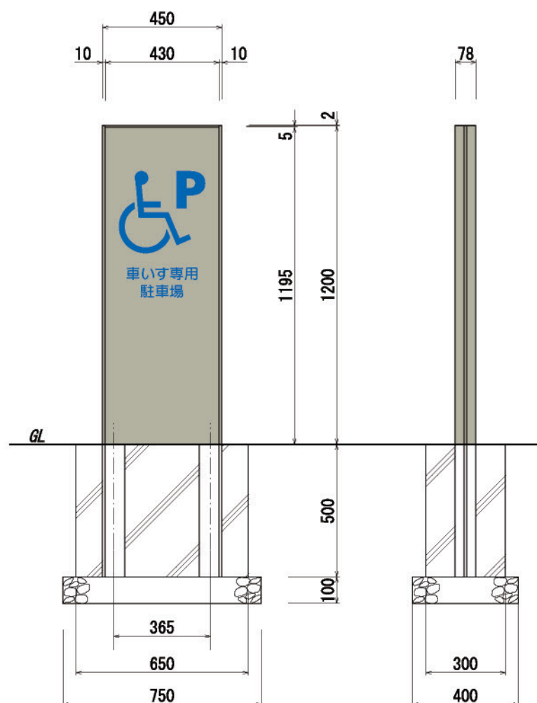
【正面図 S=1:20】
