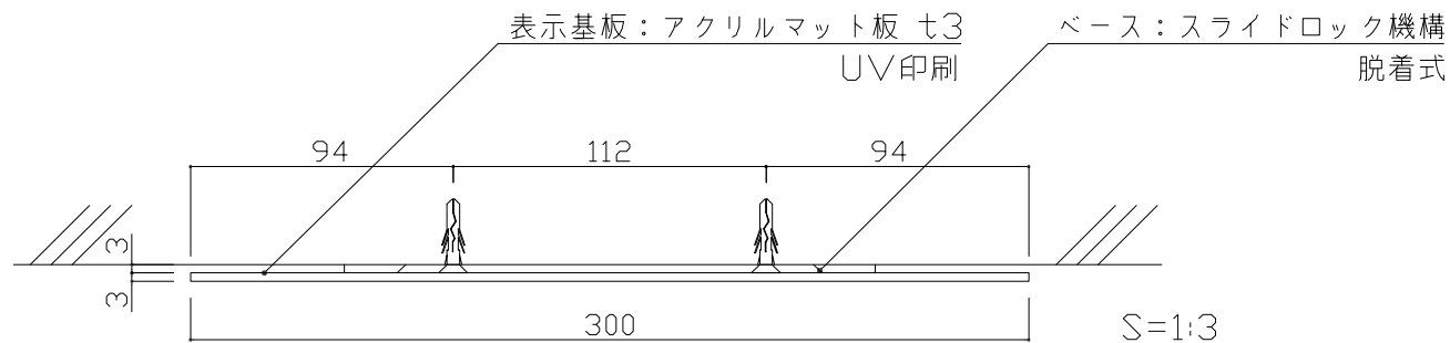
※スライドロック機構 脱着式 (ABS樹脂成形)
